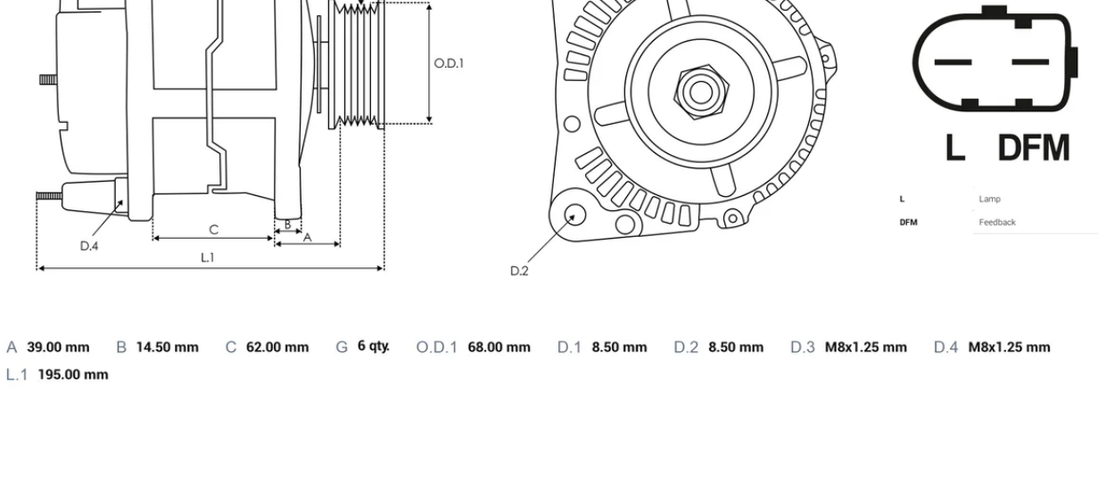
DIMENSIONS
