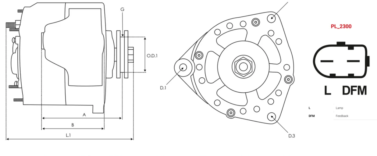
DIMENSIONS
