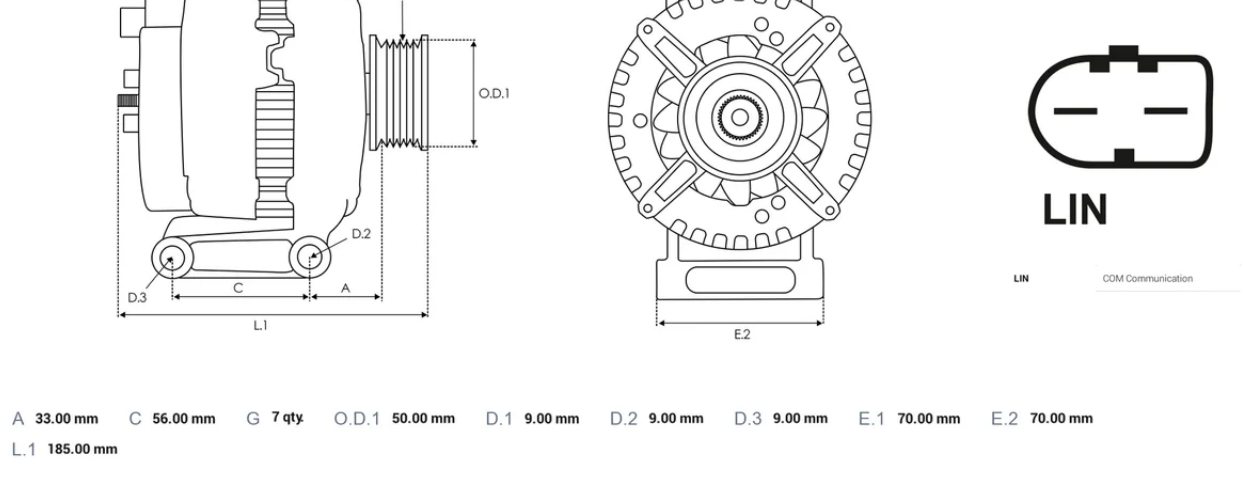
DIMENSIONS
