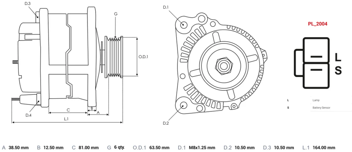
DIMENSIONS
