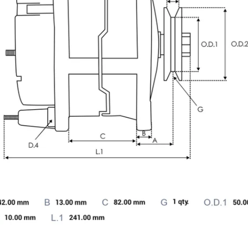
DIMENSIONS
