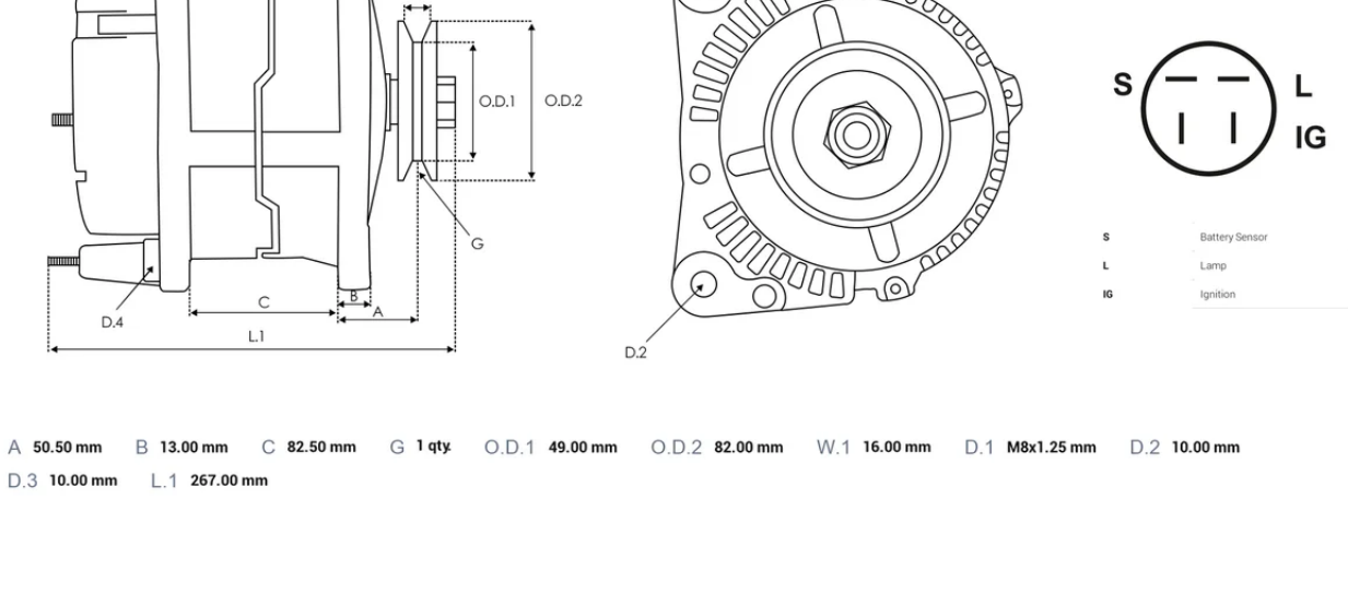
DIMENSIONS
