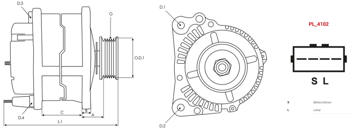
DIMENSIONS
