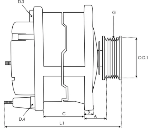
DIMENSIONS
