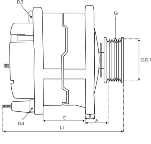
DIMENSIONS
