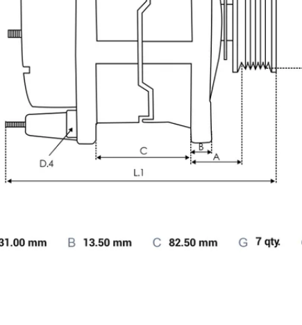
DIMENSIONS
