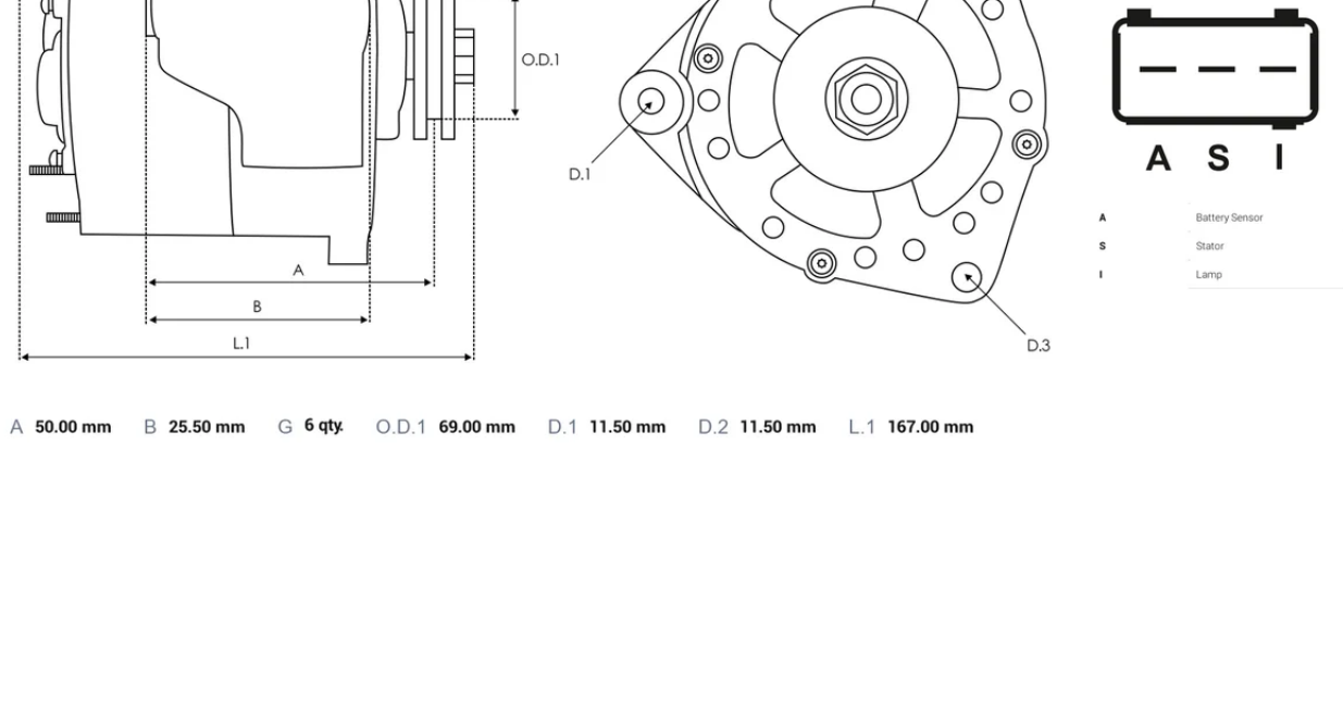
DIMENSIONS
