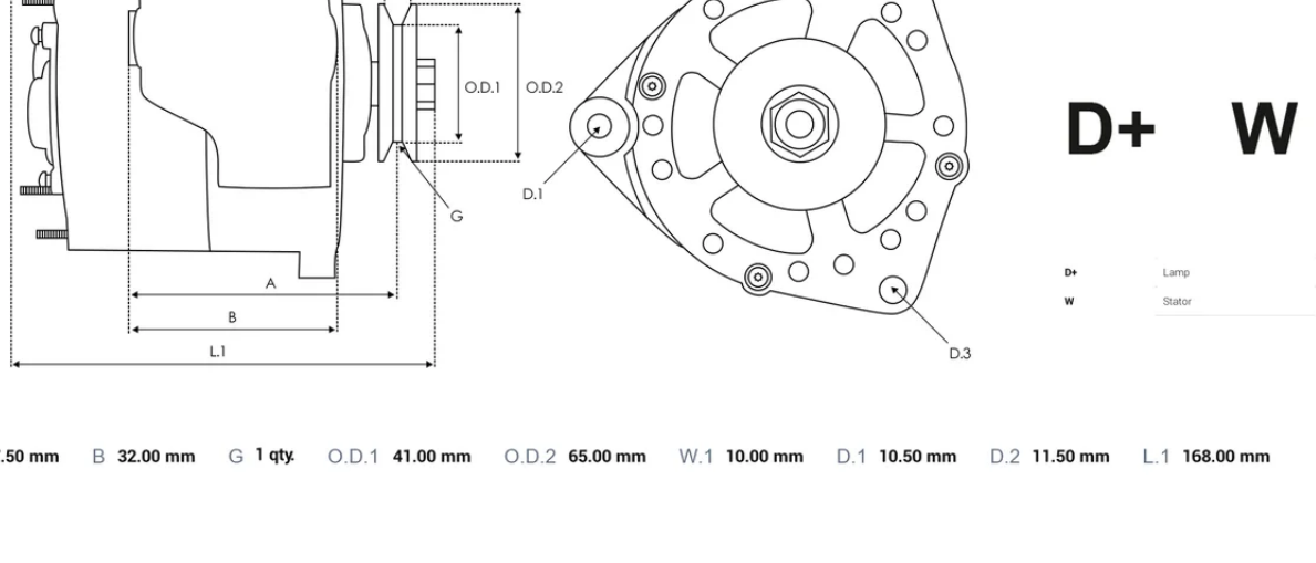
DIMENSIONS
