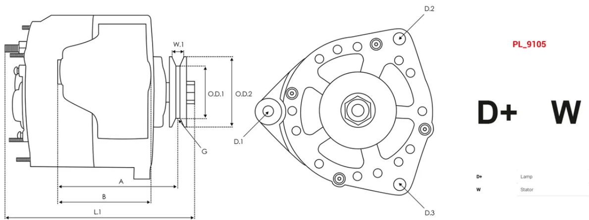
DIMENSIONS
