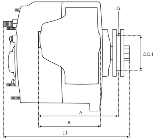
DIMENSIONS
