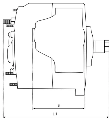
DIMENSIONS
