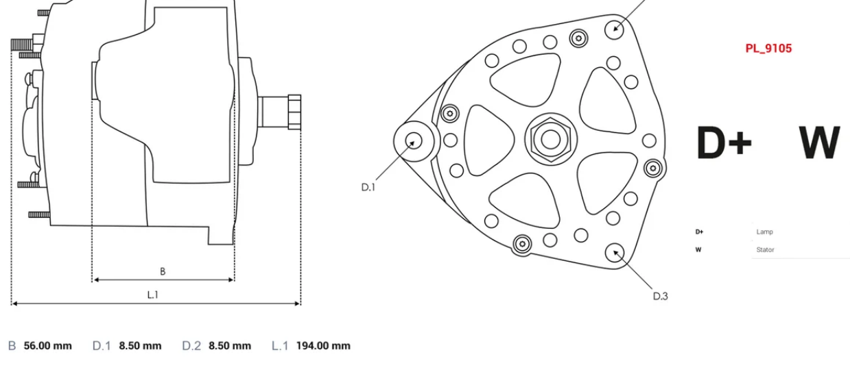
DIMENSIONS
