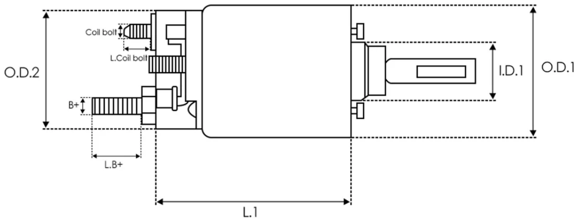
DIMENSIONS
