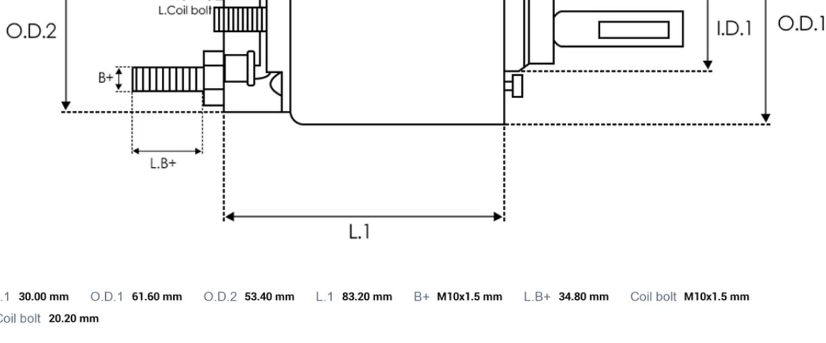
DIMENSIONS
