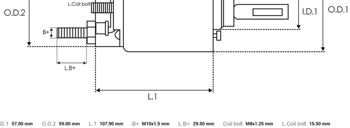
DIMENSIONS
