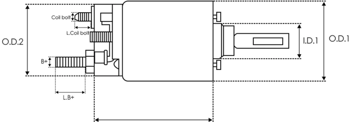
DIMENSIONS
