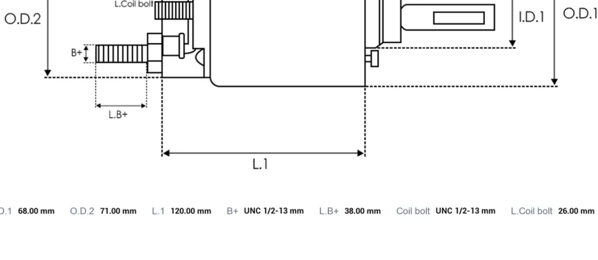
DIMENSIONS
