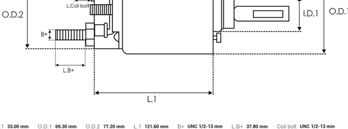
DIMENSIONS
