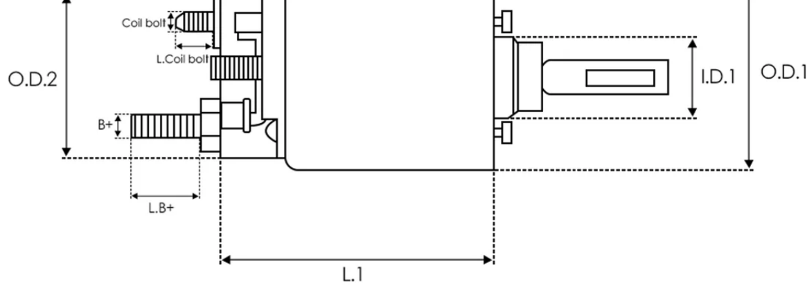
DIMENSIONS
