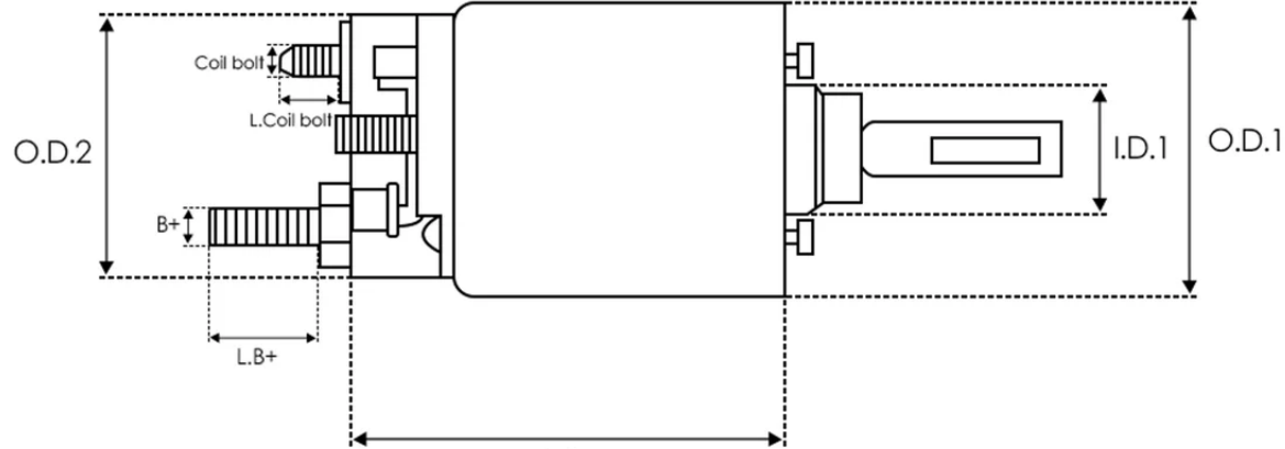
DIMENSIONS
