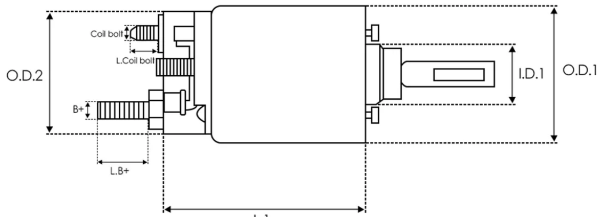
DIMENSIONS
