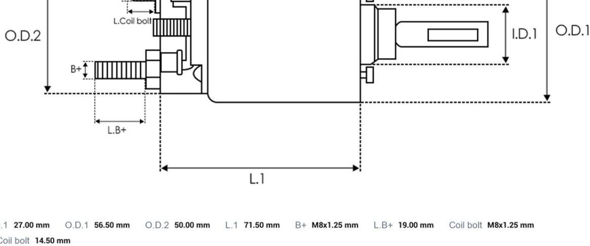
DIMENSIONS
