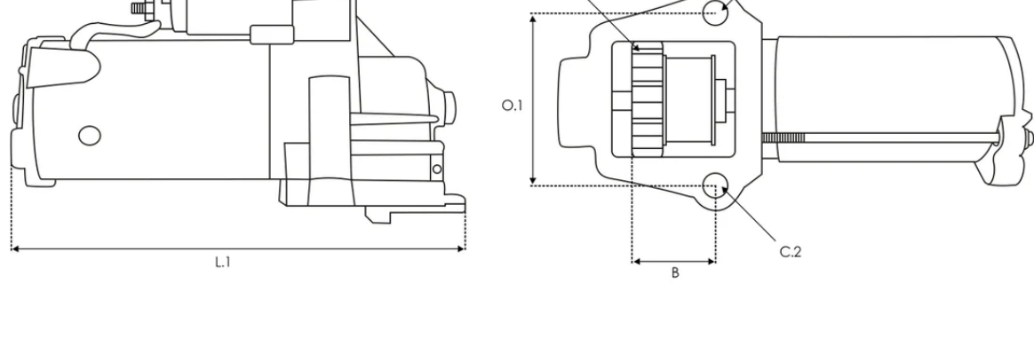
DIMENSIONS
