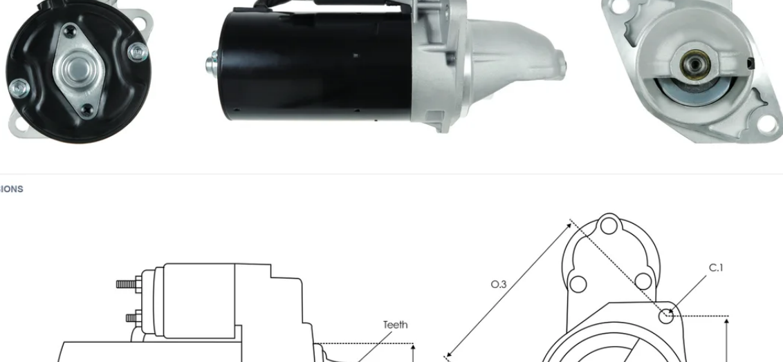
DIMENSIONS
