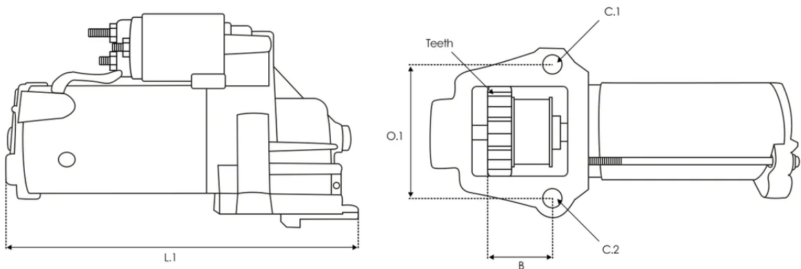
DIMENSIONS
