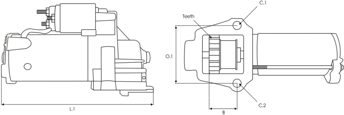
DIMENSIONS
