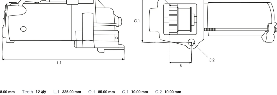
DIMENSIONS
