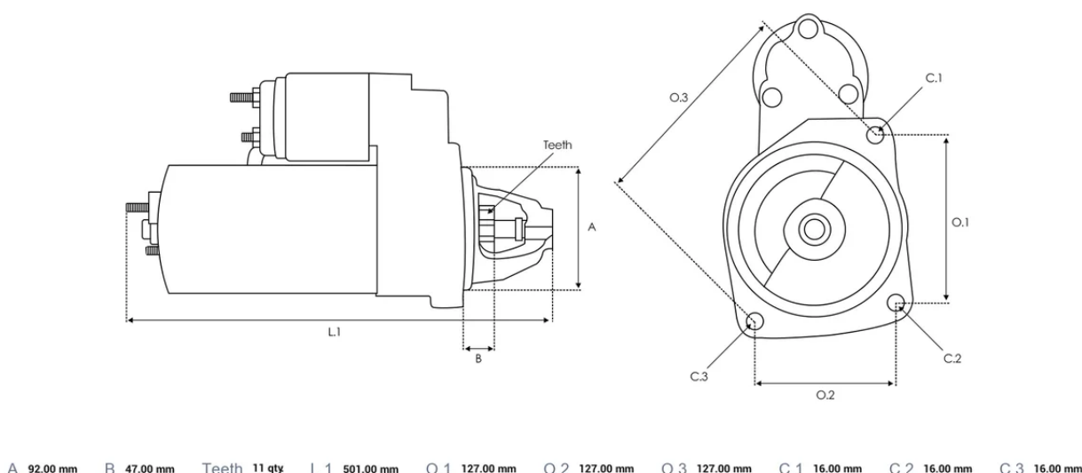
DIMENSIONS
